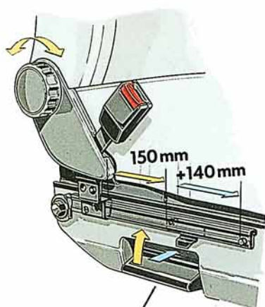
Entriegelungsgriff (Dreheinrichtung)
