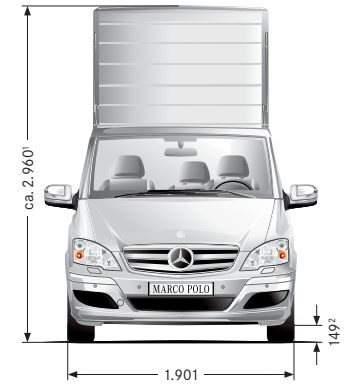
Front mit geöffnetem Aufstelldach
