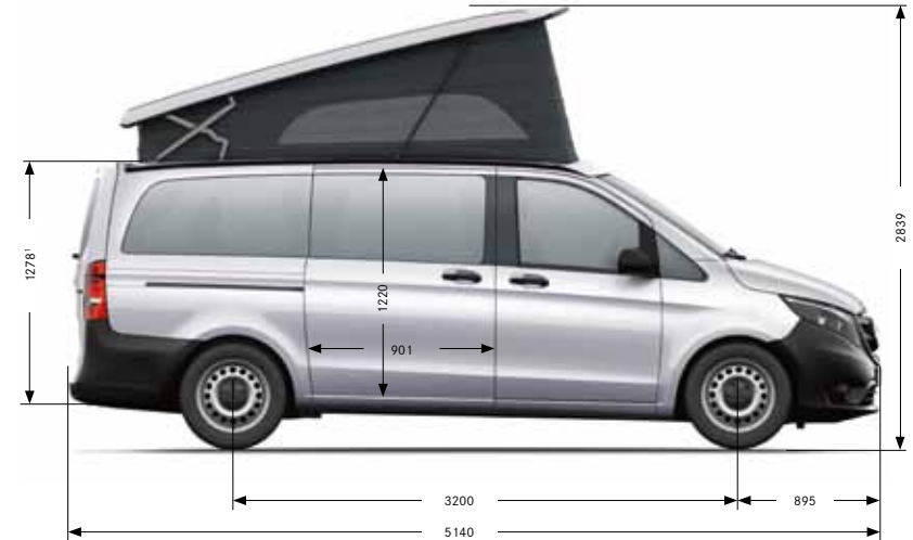
Zijaanzicht met open uitzetdak
